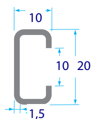
C2010Z (acier zingué) C2010X (acier inox) 0,49 kg/m
