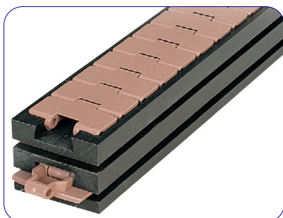
Profils droits pour chaînes biflex
