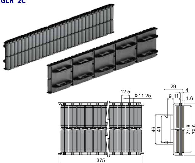
Guide latéral à galets, double hauteur FGLR 2C
