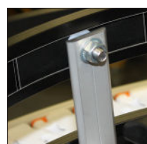
Pièce plastique FGPR FD100 en POM noir pour guides FD7-1A... en courbe
