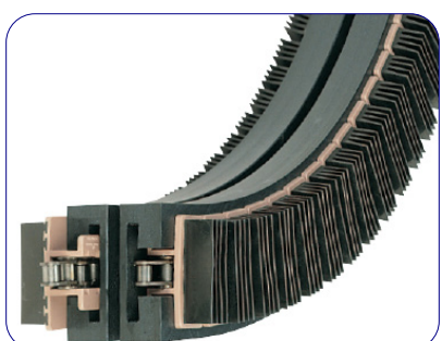
Profils droits et courbes pour chaînes «grip»
