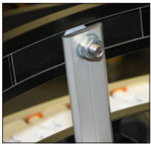
Pièce plastique FGPR FD100 en POM noir pour guides FD7-1A... en courbe
