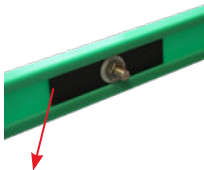
Pièce plastique FGPR FD100 en POM noir pour guides FD7-1A... en courbe
