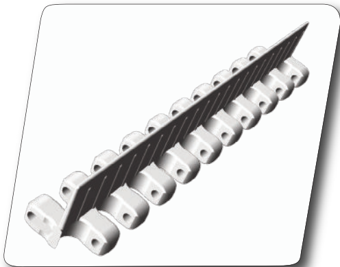
Mitnehmerhöhe 25, 50 oder 75 mm
