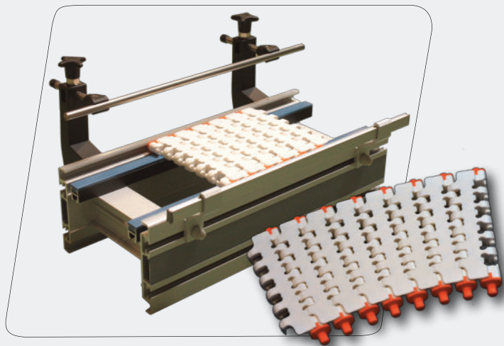
Flextoo mit modularer Kurvenmatte
