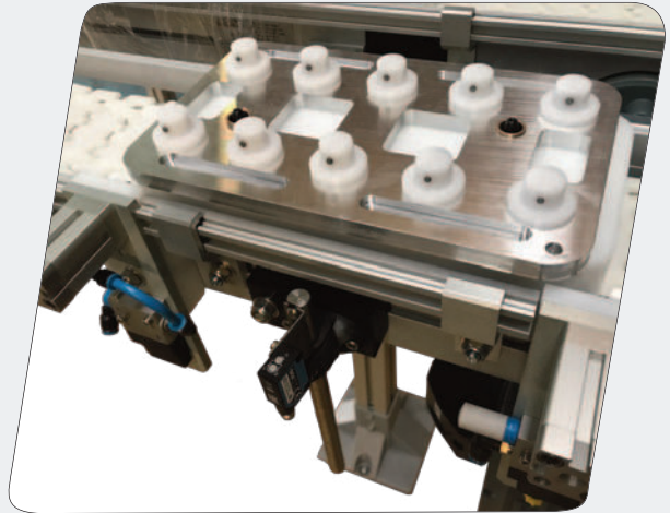
Transferts de butées porte-pièces
