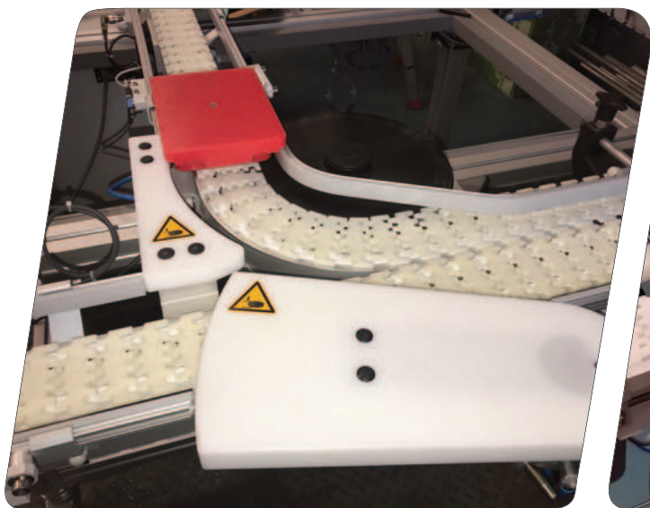
• Déviateur latéral pour changement de voie
