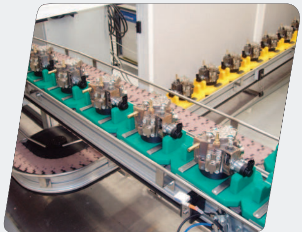
Transferts de supports de pièces mécaniques
