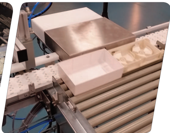
• Déviateur perpendiculaire par translation
