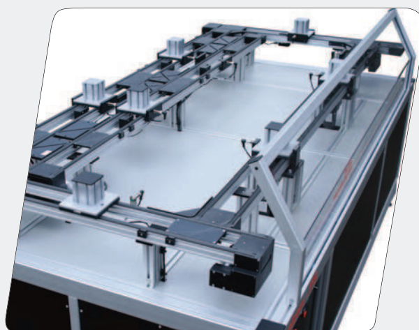
Exemple d'un transfert à palettes ITS 24V
