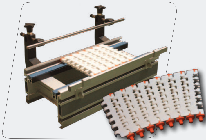
Flextoo avec tapis modulaire courbe
