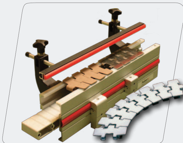
Robur avec chaîne droite ou courbe
